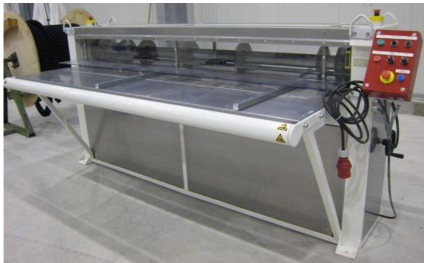
ICE-Trade Gurtschneidetisch
